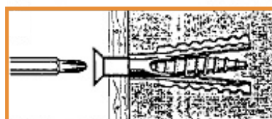
Kevytbetoni asennus
